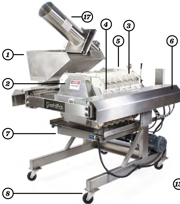
Fig 1.1: X-6 Press
